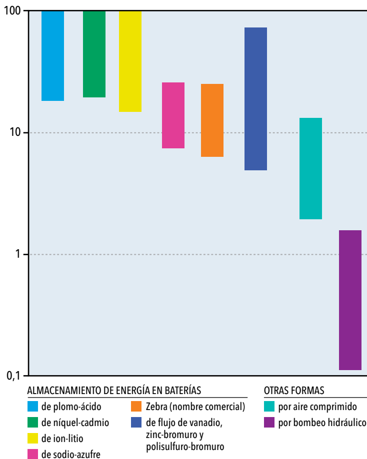
Figura 8. Costos comparativos de diferentes sistemas de almacenamiento eléctrico. Adviértase que la escala del eje vertical es logarítmica y que los costos más altos pueden ser casi mil veces mayores que los más bajos.
